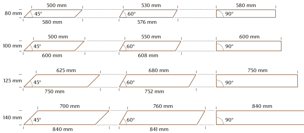
Chevron 45°
